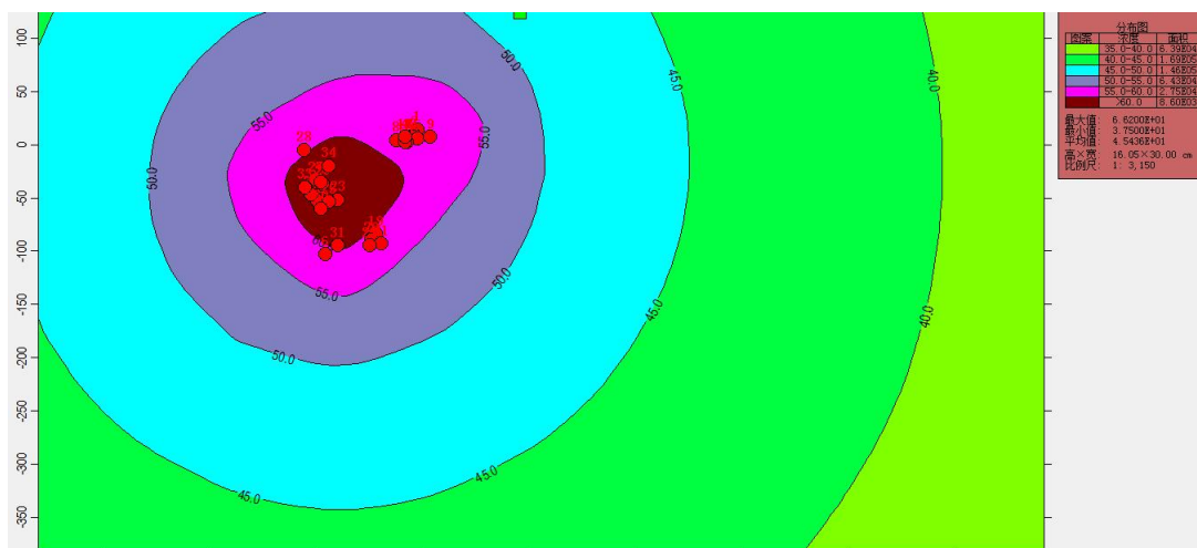
图 4-5 噪声预测图
