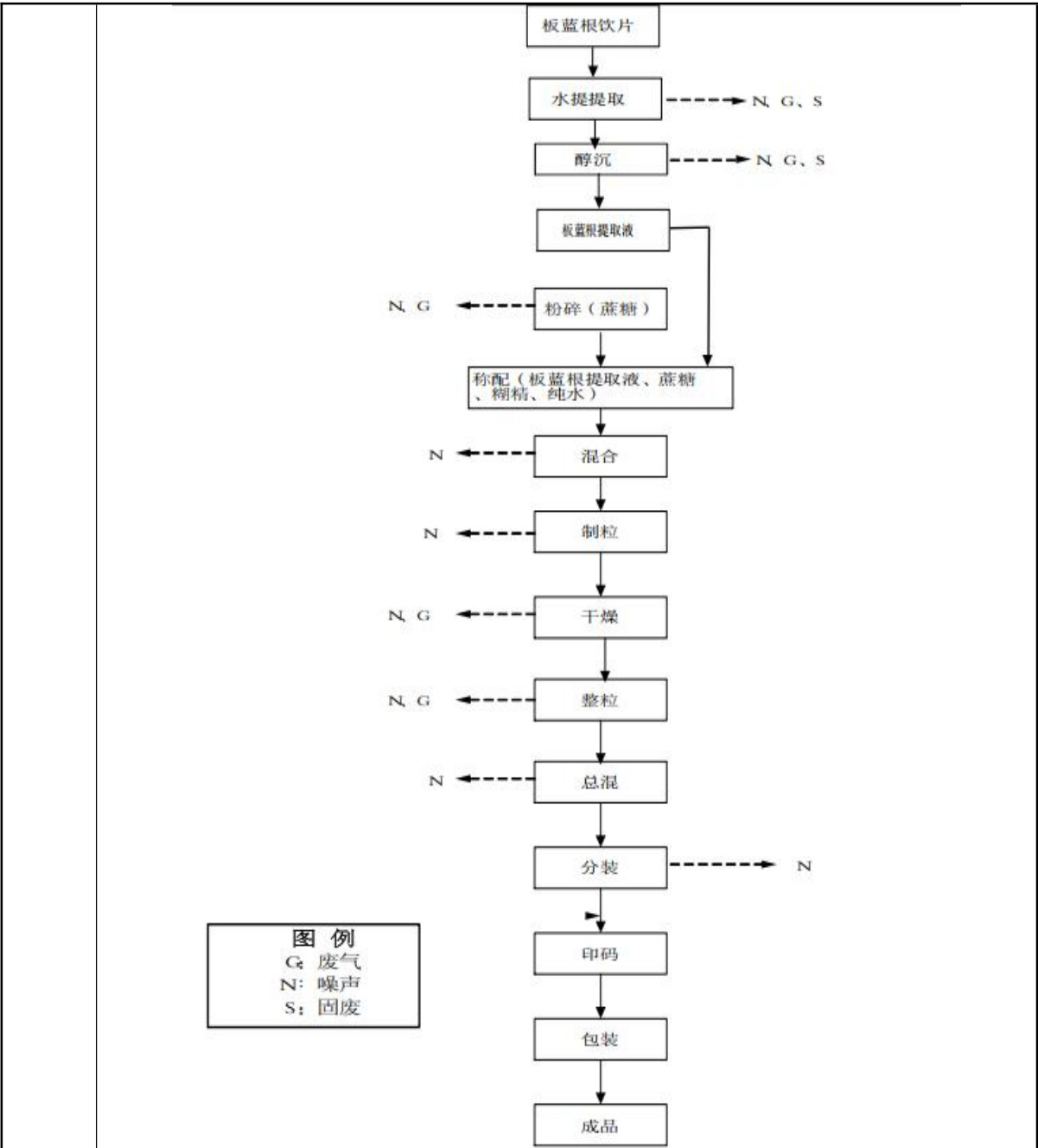
图 2-4 本项目生产工艺流程及产物环节图
